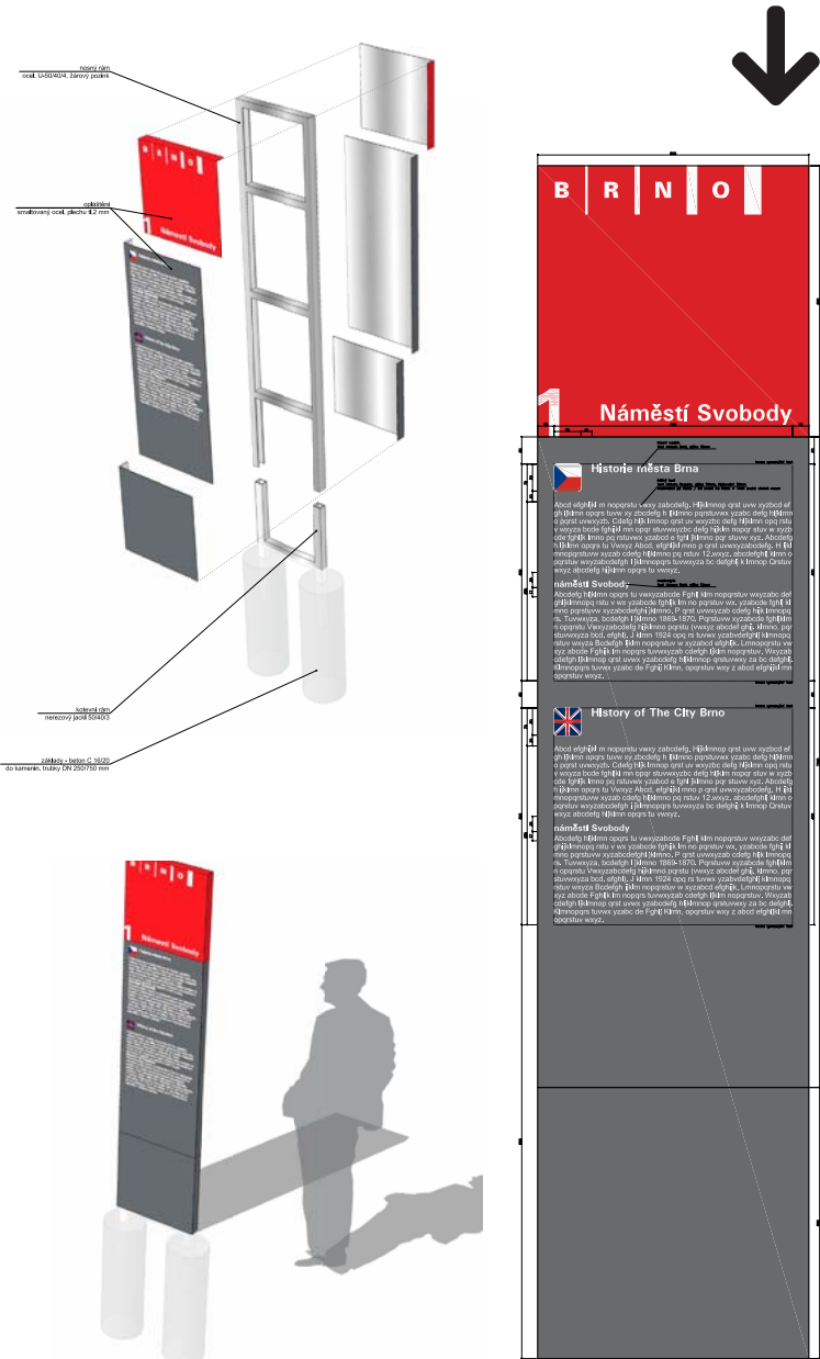
PERSPEKTIVA - KONSTRUKCE A JEDNOTLIVÉ DÍLY
