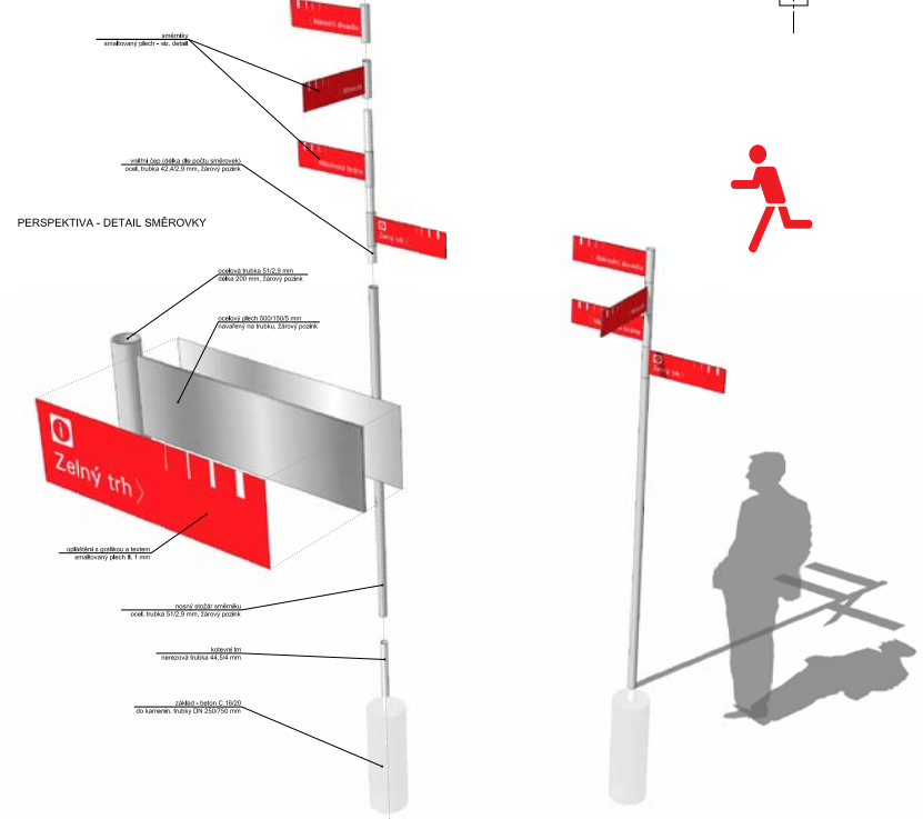
PERSPEKTIVA - JEDNOTLIVÉ DÍLY
