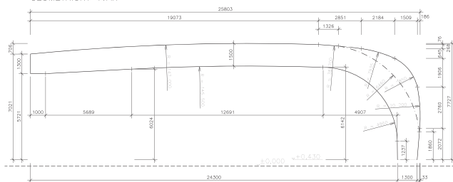
LEPENÝ NOSNÍK ČÍSLO 1 GEOMETRICKÝ TVAR
