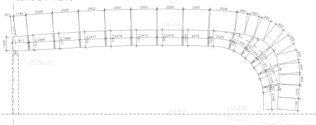
LEPENÝ NOSNÍK ČÍSLO 1 ROZMÍSTĚNÍ VAZNIC
