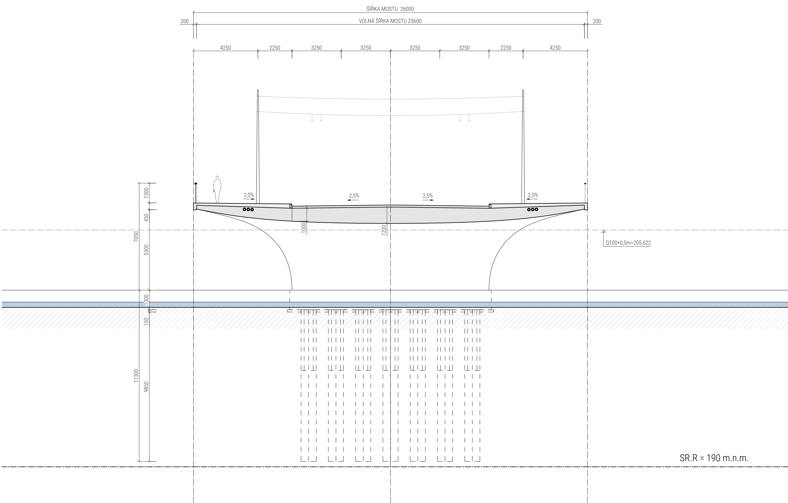
Řez vrcholem mostu 1:150
