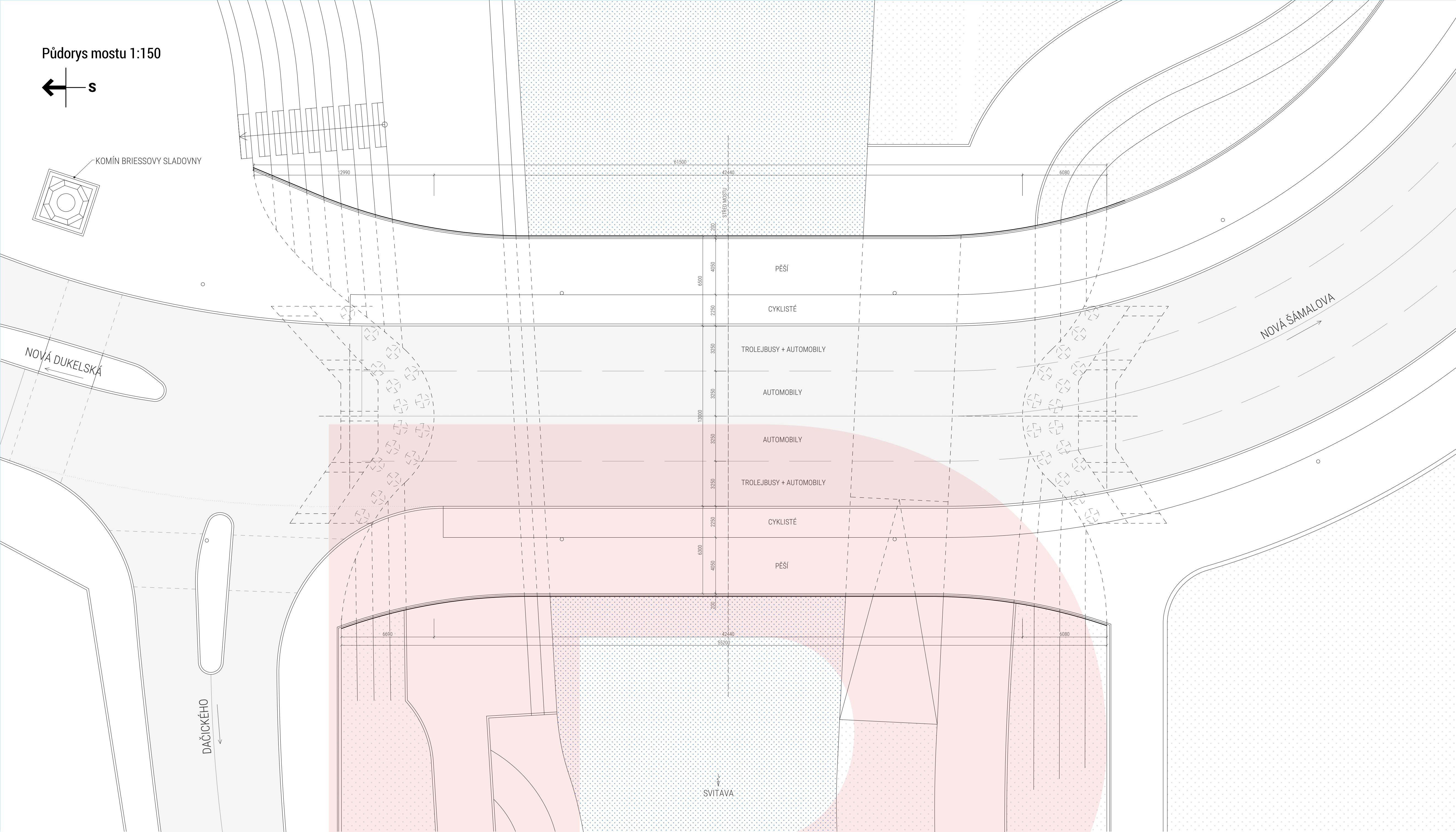
Podélný řez mostem 1:150
