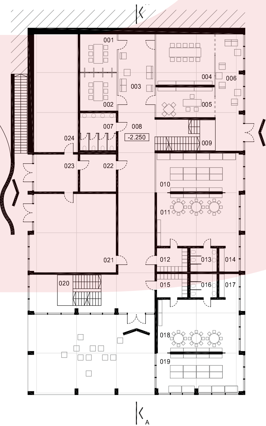
PATRO -1 1:250
