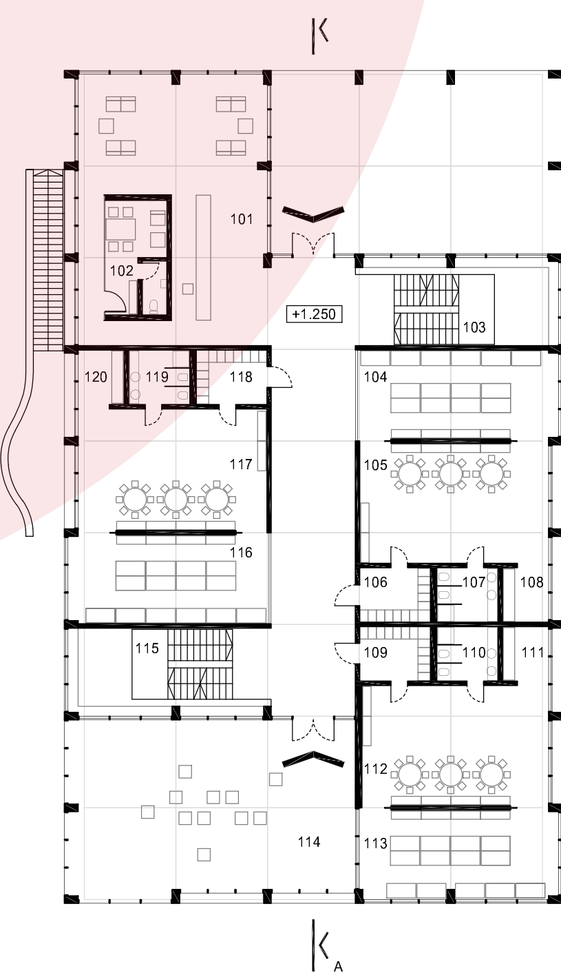
PATRO 1 1:250
