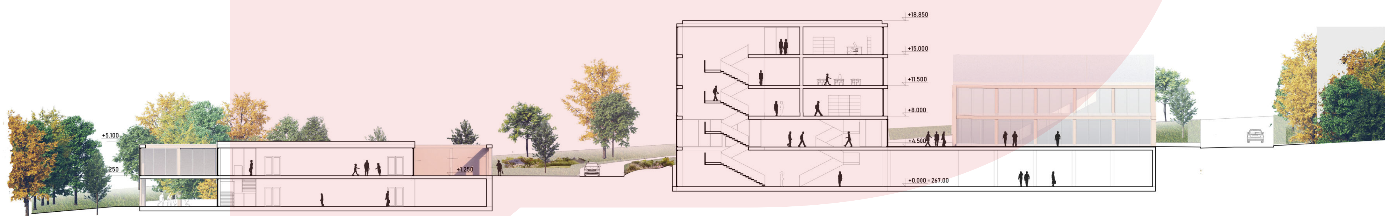
VÝKRES ŘEZU A-A 1:250
